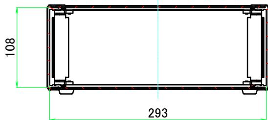
B-B ( 1 : 5 )
