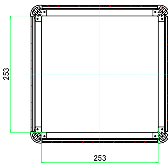
C-C ( 1 : 5 )
