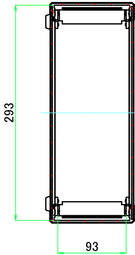
A-A ( 1 : 5 )
